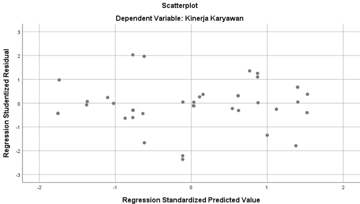
Gambar 1. Uji Heteroskedastisitas
